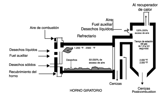
Figura 9.23: Horno rotatorio.
