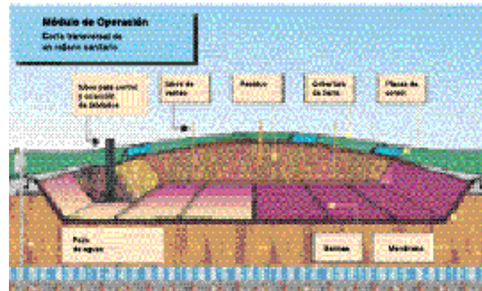
Figura 10.1. Componentes de un Relleno Sanitario.
