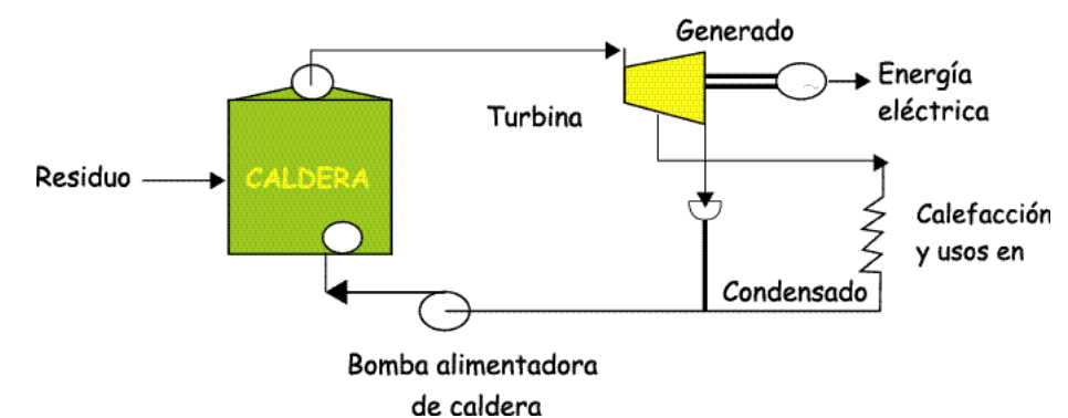
Figura 9.24: Recuperación de energía usando turbina a vapor.
