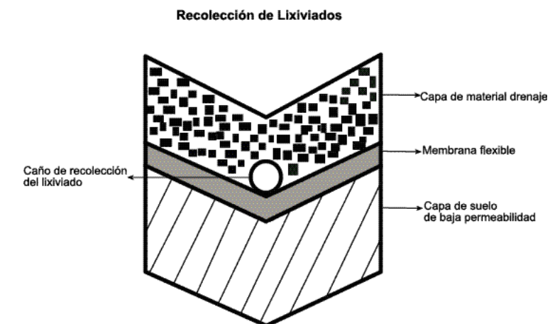
Figura 10.5. Sistema de recolección de lixiviado.
