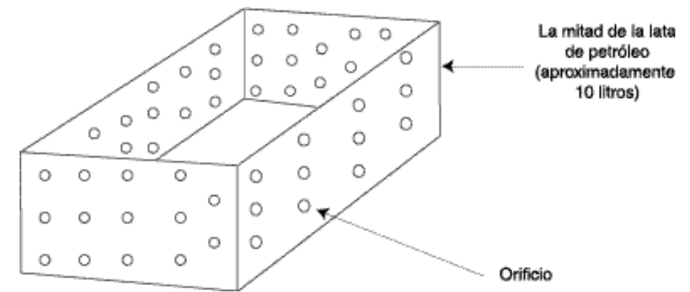
Figura 15.2. Diagrama de receptáculos para determinación de humedad.
