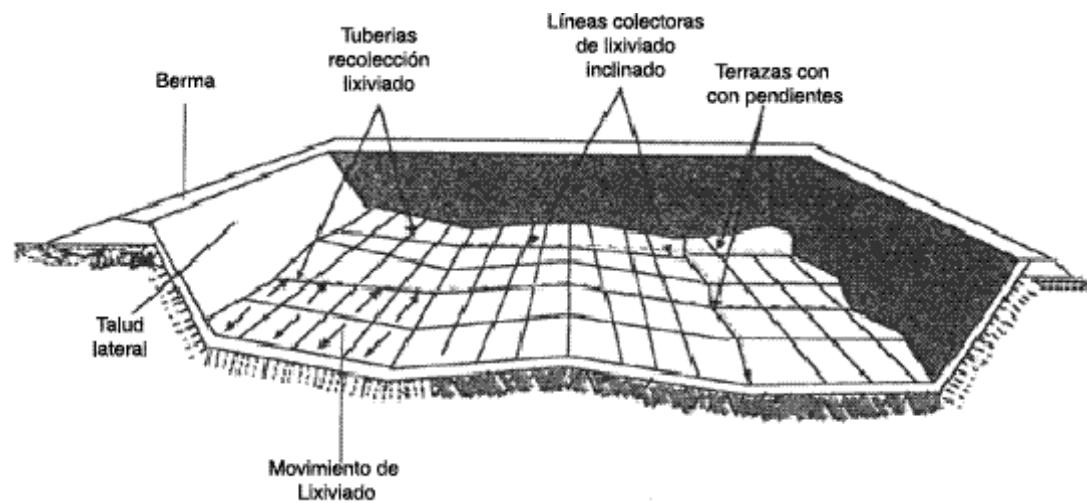
Figura 10.6. Sistema de pendientes para la localización de tubos de lixiviados.
